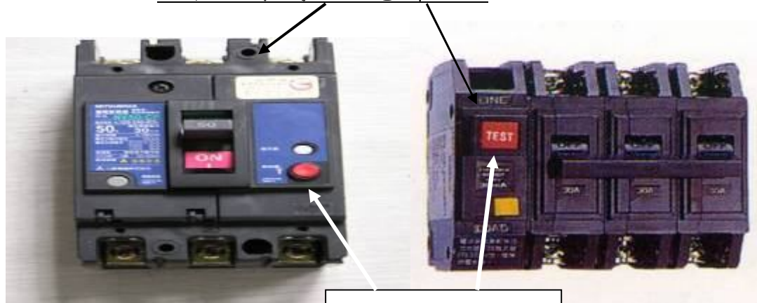
漏電斷路器測試鈕
